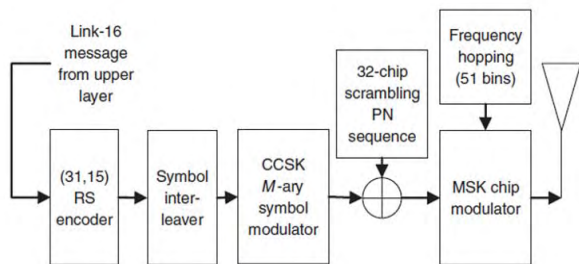
그림 2. Link-16 송신시스템 모델[2]
